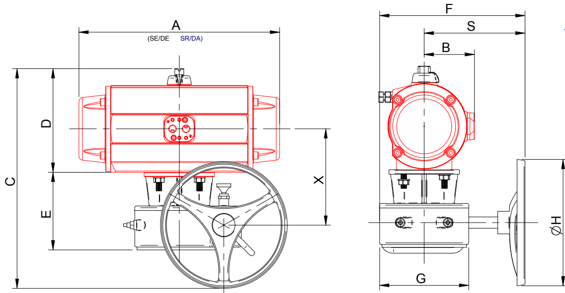
DIMENSIONES DEL CONJUNTO ACTUADOR + REDUCTOR
